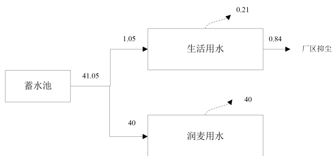
图 2 项目采暖季水平衡图 (m 3 /d)
