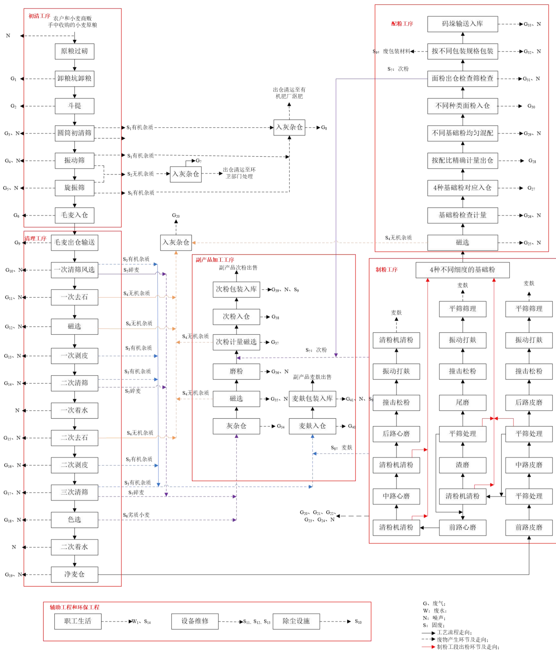
图 4 小麦加工生产工艺流程及产污环节示意图
