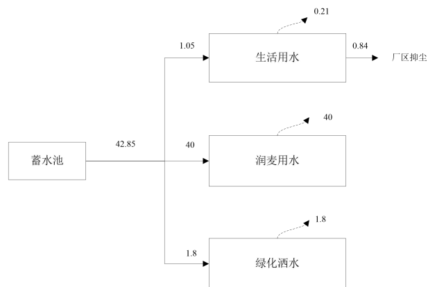
图 1 项目非采暖季水平衡图 ( \text{m}^3/\text{d} )
